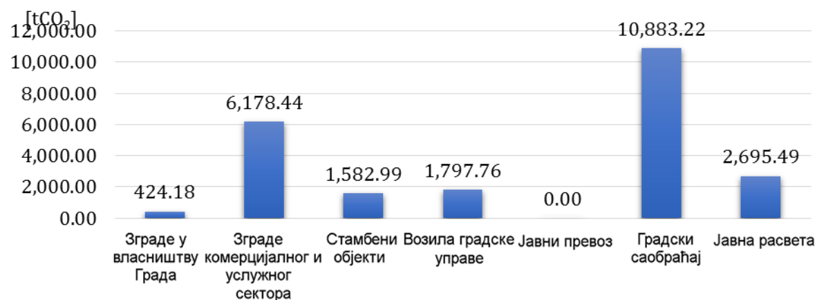
Слика 15 – Укупна емисија CO 2 према подсекторима Чајетина
