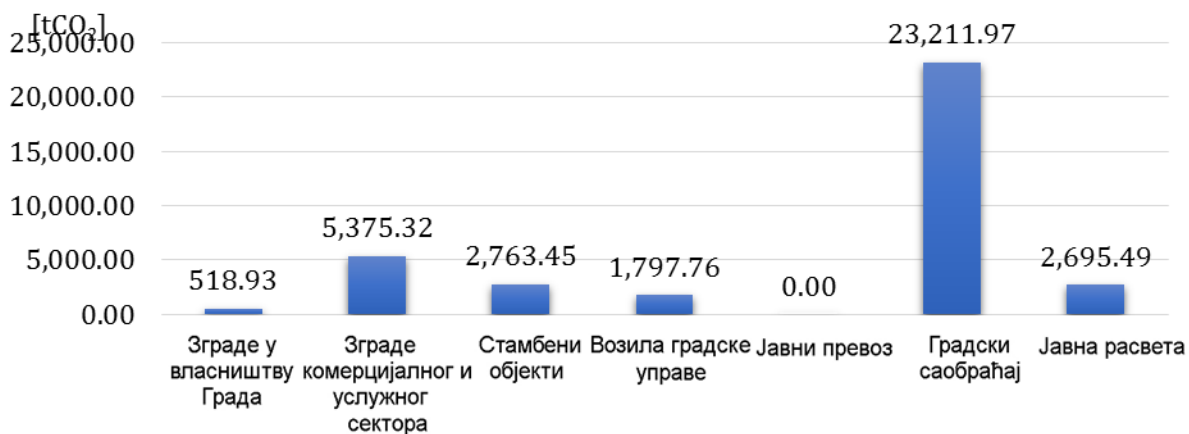
Слика 9 – Укупна емисија CO 2 према подсекторима Прибој
