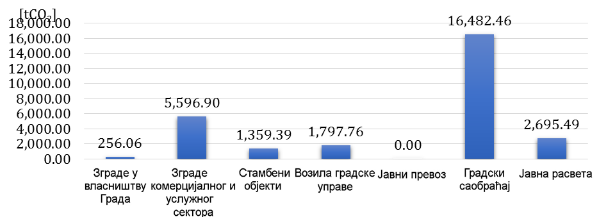
Слика 19 – Укупна емисија CO 2 према подсекторима Ариље
